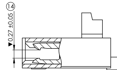
剖面A-A
